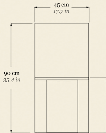
vue de dos
